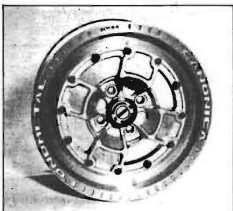
CANORALLY 1 - 4 fori scomponibile in 2 pezzi per tutte le auto italiane e straniere nelle misure: 5x13 5 1/2x13 - 6x13 - 7x13 - 5 1/2x14 - 6x14 - 6x15
